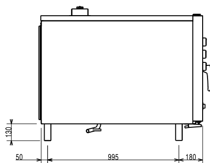
Oldalnézet
